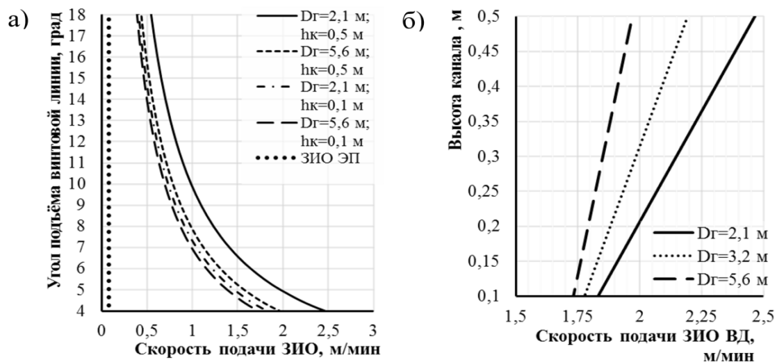
Рисунок 1. Зависимость скорости подачи ЗИО от угла подъёма винтовой линии (а) и высоты канал (б).
