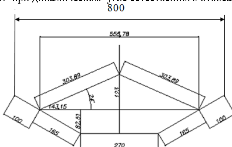
Рис. 1. Модель расположения груза на ленте в сечении
