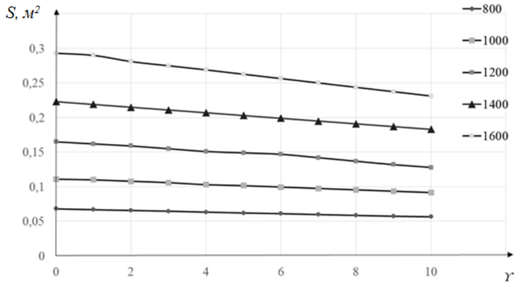
Рис. 3. Зависимость площади сечения груза на ленте от угла наклона роlikоопоры
