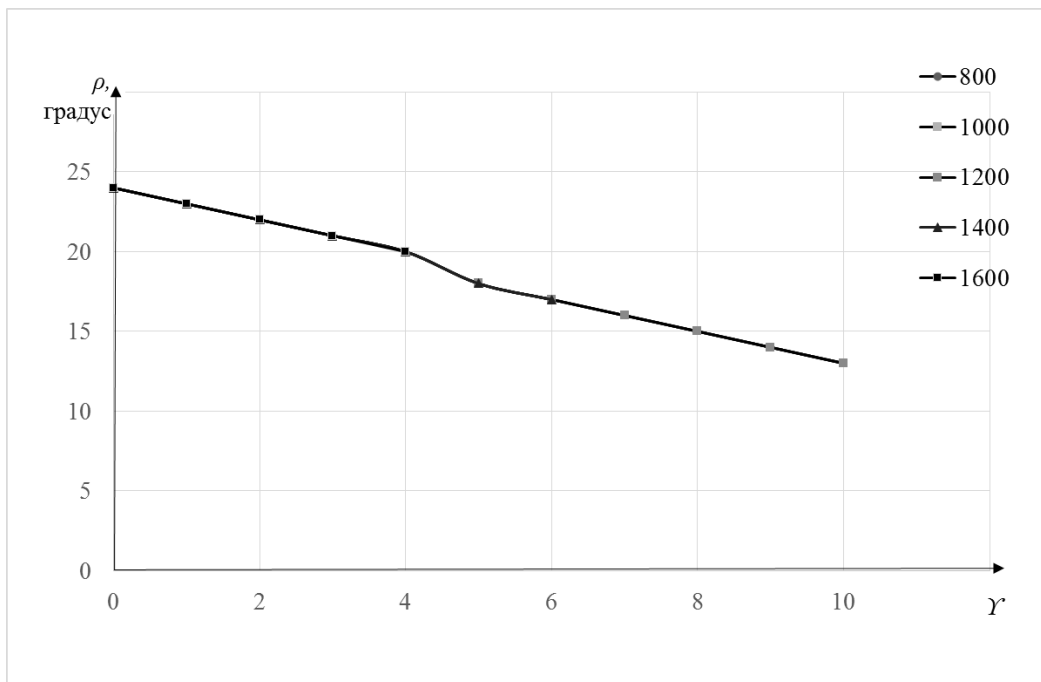
Рис. 4. Зависимость динамического угла естественного откоса от угла наклона роlikоопоры
