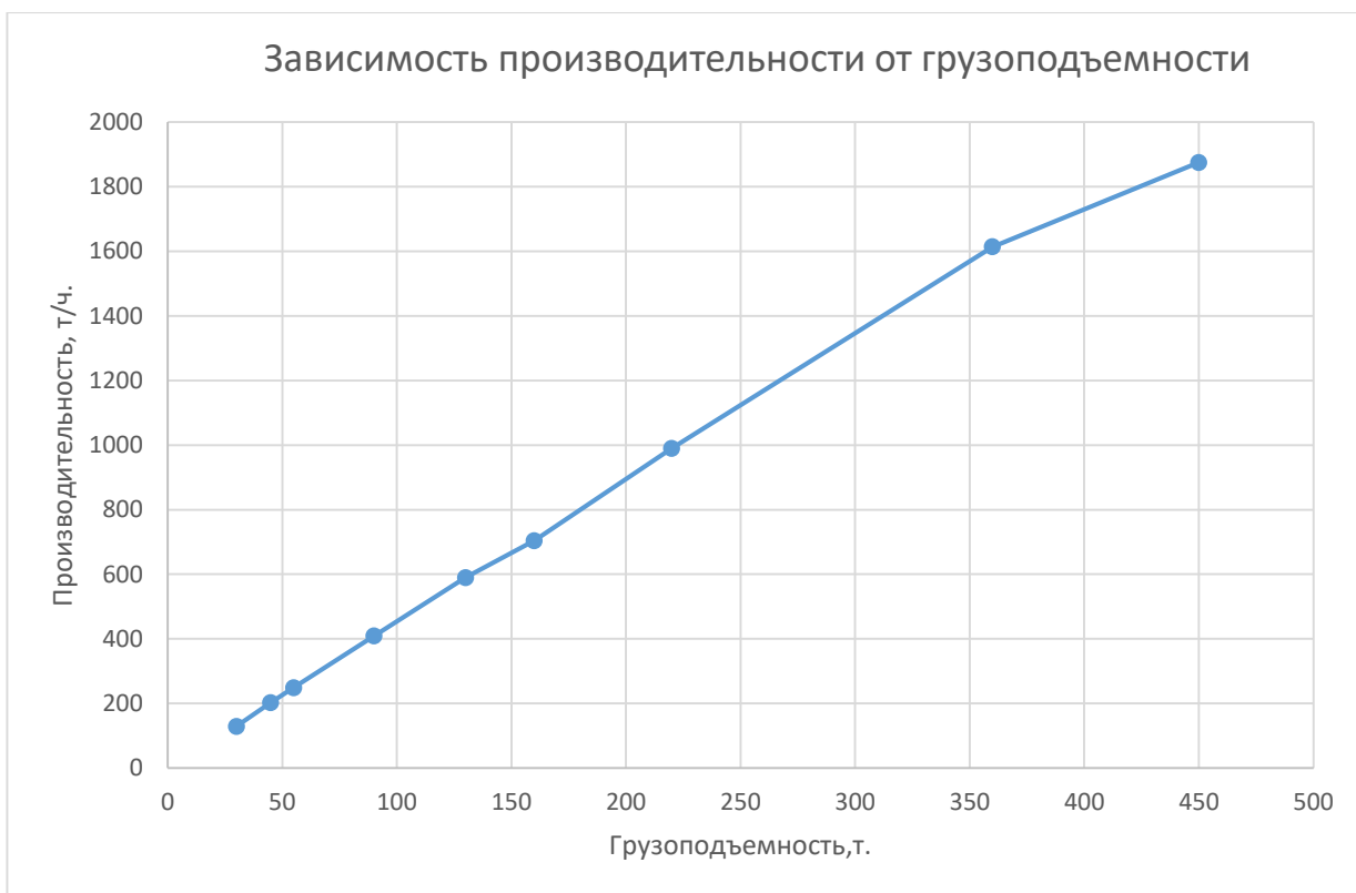
Рис.3 Зависимость производительности от грузоподъемности автосамосвалов
