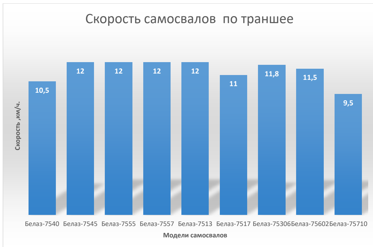
Рис. 1. Скорость движения автосамосвалов вверх по траншее (средневзвешенный уклон 70 ‰)
