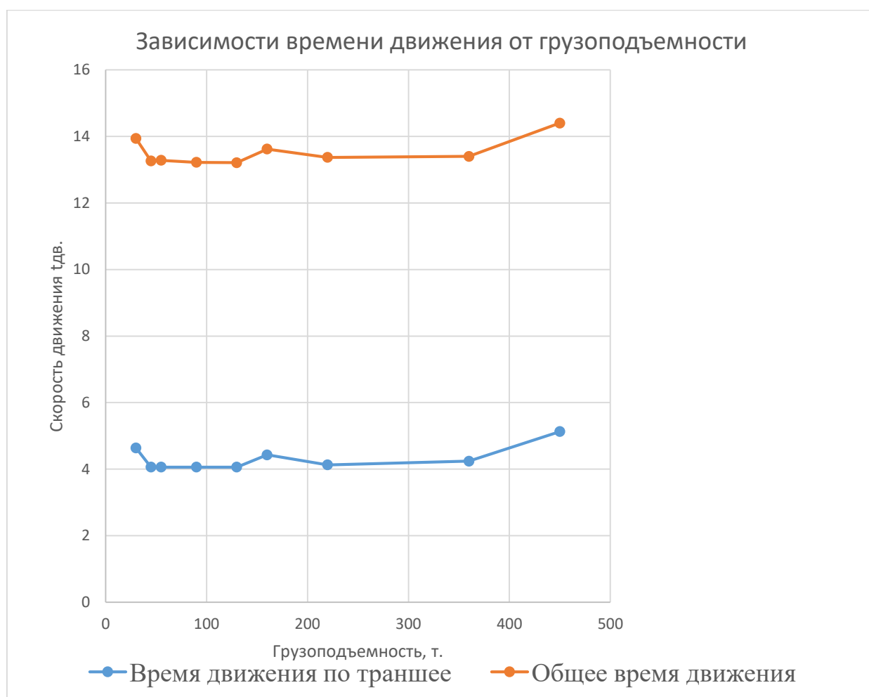
Рис. 2. Время движения автосамосвалов по траншее на подъем и общее время движения за рейс
