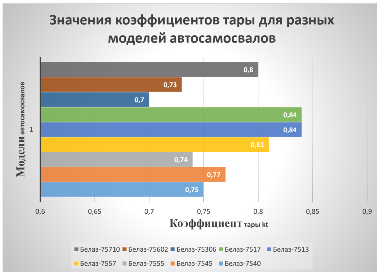
Рис. 4 Значение коэффициента тары для базовых моделей автосамосвалов
