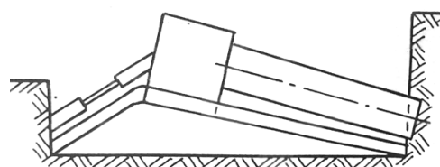
Рис. 3. Вариант неустойчивого состояния буровой машины «Ричмонд»
