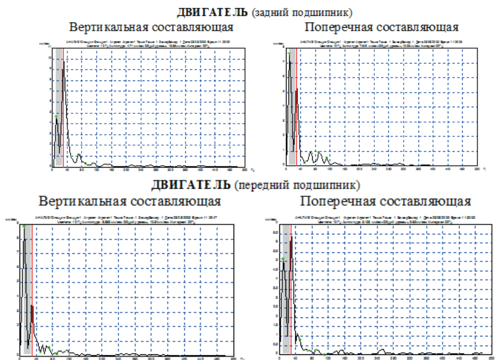
Рисунок 6. Интенсивность вибрации на двигателе скребкового конвейера Figure 6. Vibration intensity on the scraper conveyor motor
