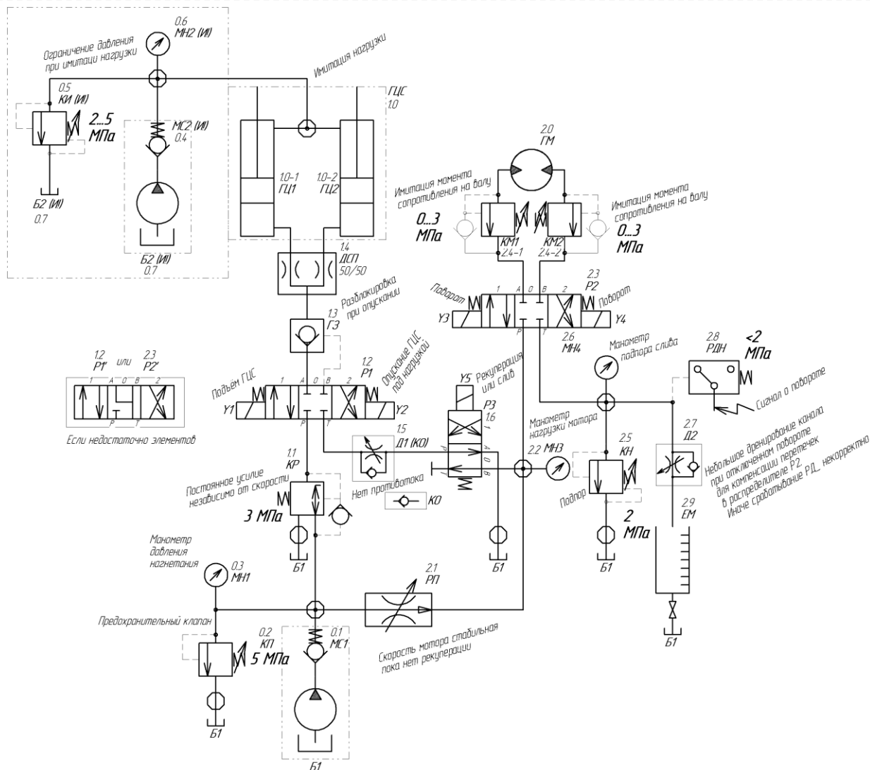
Рис. 3. Гидросхема конечная с электроуправлением и имитацией перетечек Fig. 3. Final hydraulic circuit with electrical control and imitation of leaks
