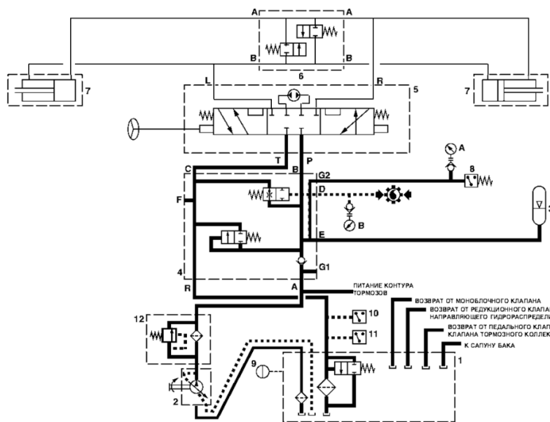
Рис. 1. Гидравлическая схема системы рулевого управления Terex TR 100: 1 – бак рабочей жидкости рулевого управления и тормозов, 2 – насос рулевого механизма; 3 – гидроаккумулятор; 4 – клапан гидроаккумулятора; 5 – клапан рулевого управления; 6 – разгрузочный клапан двустороннего действия; 7 – цилиндр рулевого механизма; 8 – реле давления масла; 9 – реле уровня масла; 10 – реле давления масла; 11 – реле температуры масла; 11 – фильтр рулевого управления Fig. 1. Hydraulic diagram of the Terex TR 100 steering system: 1 – steering and brake working fluid tank, 2 – steering gear pump; 3 – hydraulic accumulator; 4 – hydraulic accumulator valve; 5 – steering valve; 6 – double-acting unloading valve; 7 – steering cylinder; 8 – oil pressure switch; 9 – oil level switch; 10 – oil pressure switch; 11 – oil temperature switch; 11 – steering filter
