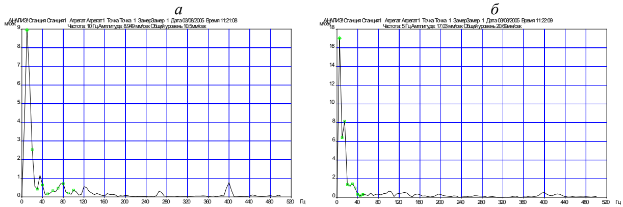
Рис. 3. Интенсивность вибрации на заднем подшипнике гидродвигателя ленточного перегружателя (а) и на выходном валу редуктора (б)
