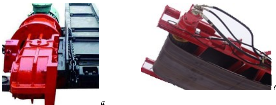
Рис. 2. Привода скребкового конвейера (а) и ленточного перегружателя (б) комплекса Superior Highwall Miners
