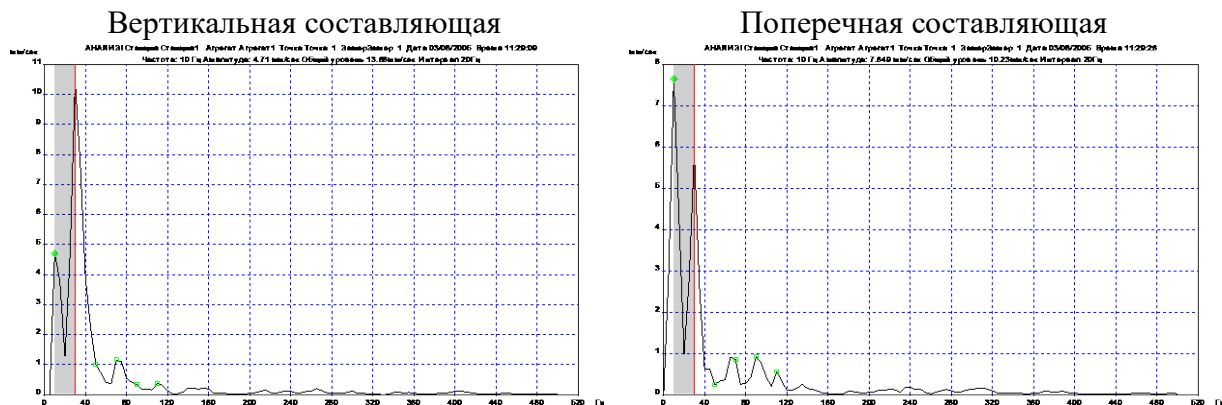
Рис. 4. Интенсивность вибрации на двигателе скребкового конвейера
