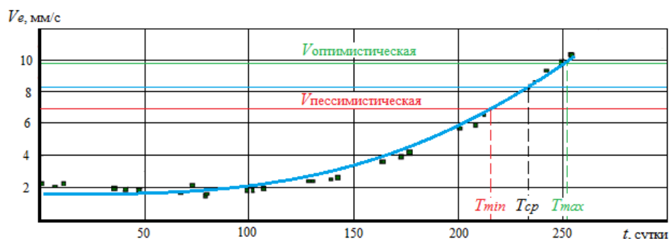
Рис. 5. Изменение СКЗ виброскорости во времени при дисбалансе выходного вала редуктора
