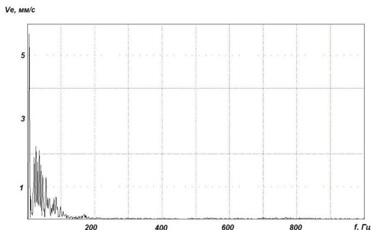
Рис. 4. Недопустимое биение и износ ременной передачи привода компрессора ПК-1,7
