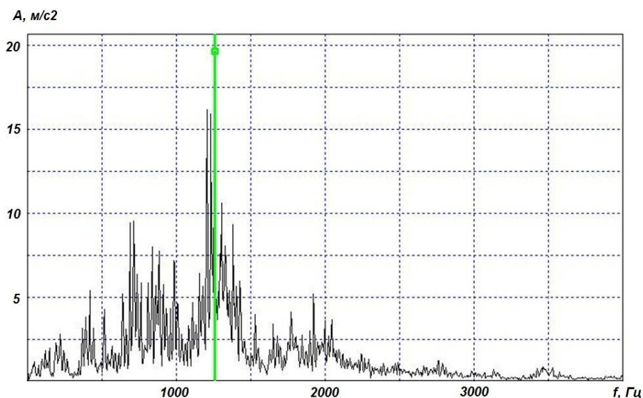
Рис. 3. Спектр по параметру виброускорения, записанный на подшипниковой опоре компрессора ПК-1,7. Общий уровень A=142,1 м/с² Fig. 3. The spectrum according to the vibration acceleration parameter, recorded on bearing support of the PK-1.7 compressor. General level A=142.1 m/s²
