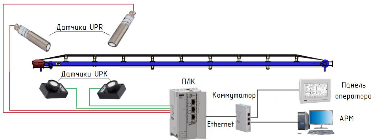
Рис. 4. Структурная схема УОПП, реализованная с использованием УЗ датчиков серий UPR и UPK
