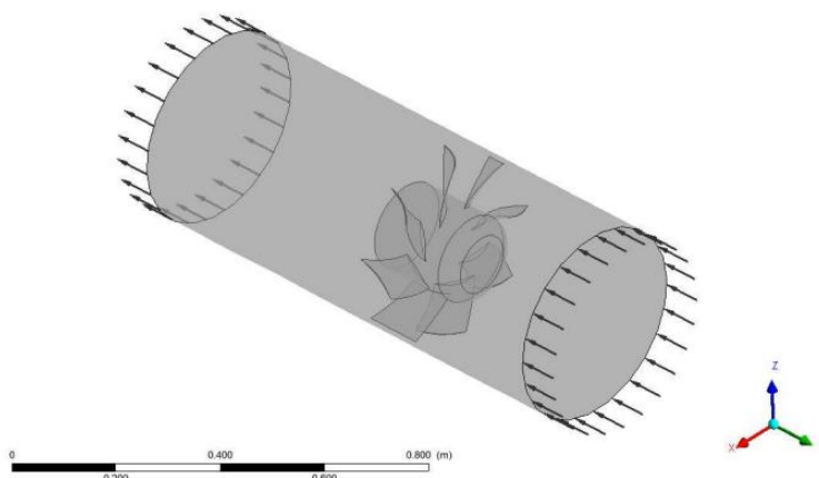
Рисунок 2. Движение воздуха в трубе [7]
