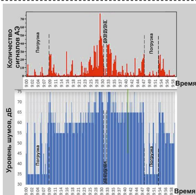
Рис. 14. Активность АЭ сигналов и уровень шумов за 1 час (датчик № 8)
