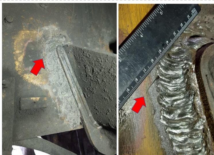
Рис. 12. Дефект в сварном шве опоры двигателя (датчик № 12) Fig. 12. Defect in the weld seam of the engine mount (sensor No. 12)
