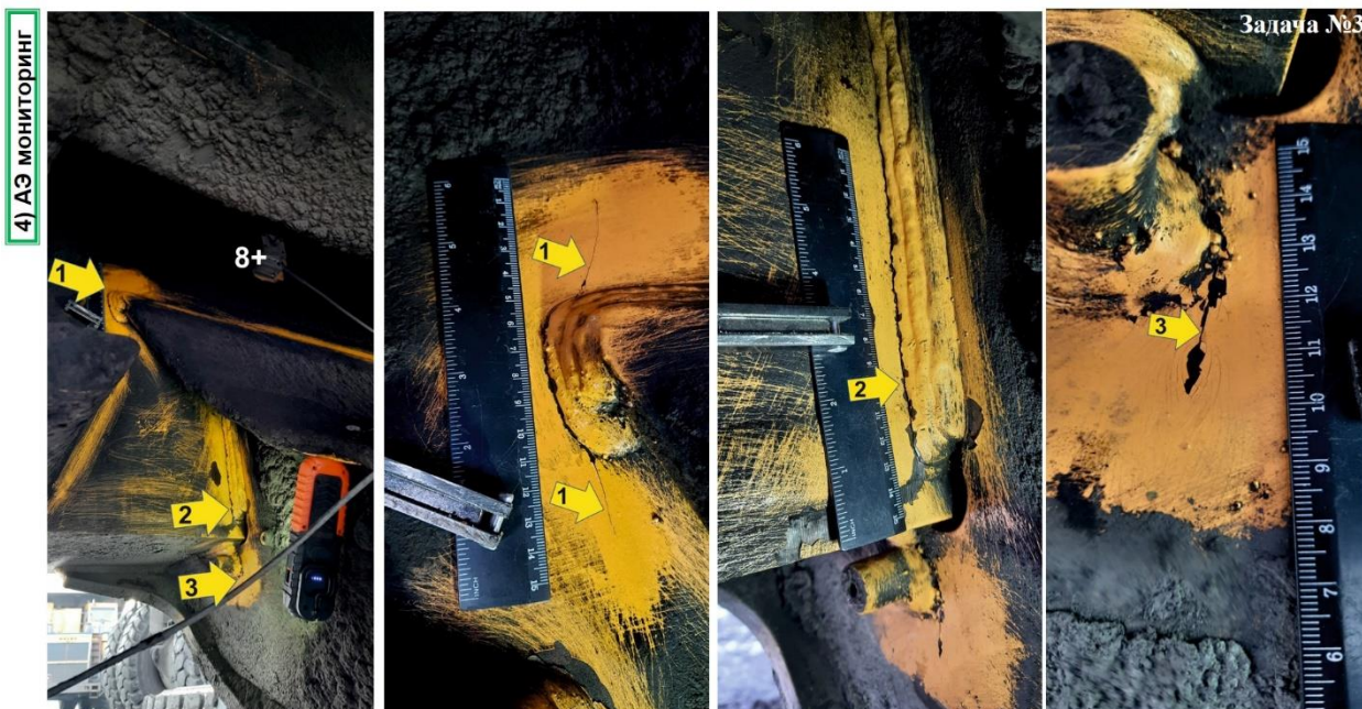
Рис. 10. Дефекты рамы, в районе 2-ой перемычки (датчик № 8) Fig. 10. Frame defects, in the area of the 2nd jumper (sensor No. 8)
