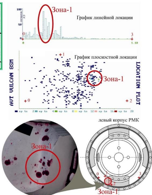
Рис. 5. Зоны повышенной активности АЭ сигналов на корпусах РМК
