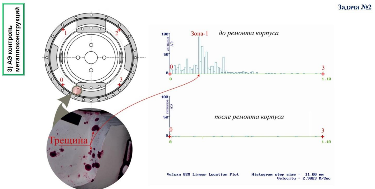
Рис. 6. Зоны повышенной активности АЭ сигналов до и после ремонта Fig. 6. Zones of increased activity of AE signals before and after renovation
