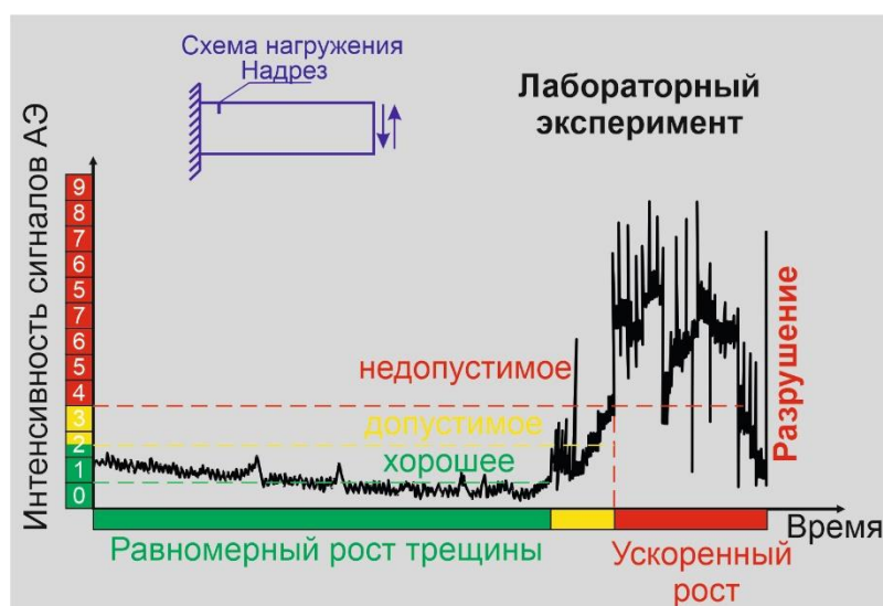
Рис. 2. Испытания с АЭ контролем при циклическом изгибе надрезанного образца
