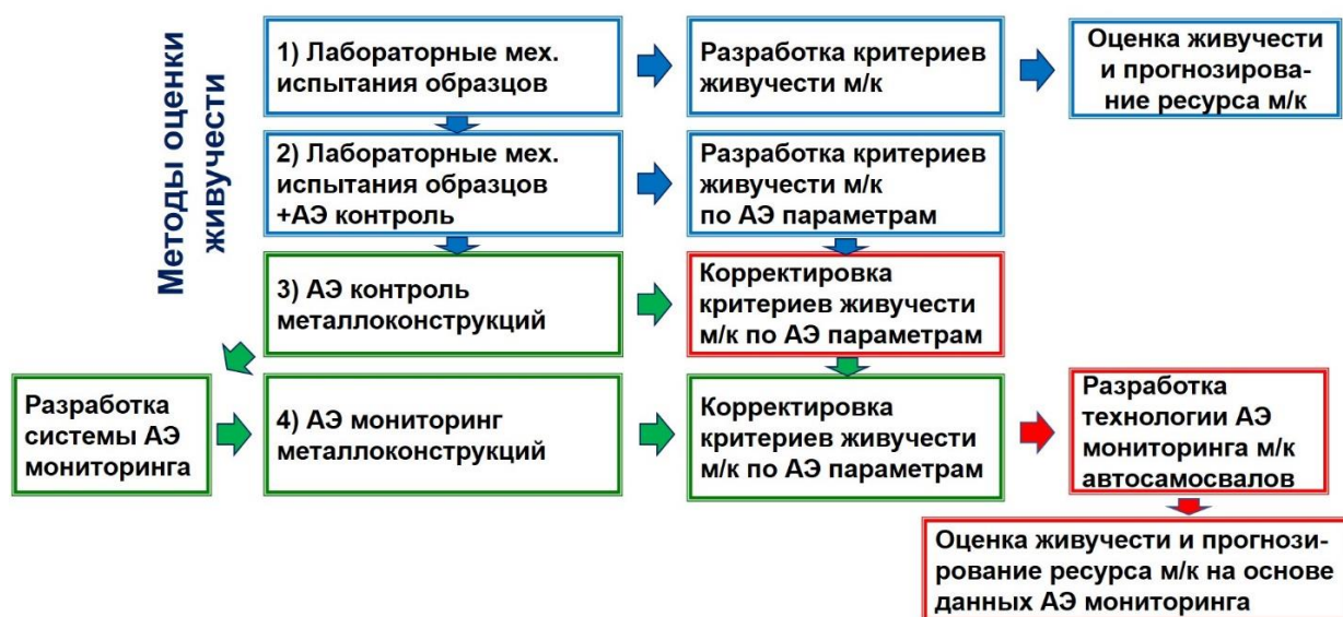
Рис. 1. Этапы разработки критериев живучести на основе АЭ метода
