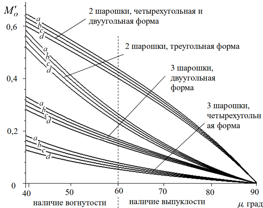
Рис. 2. Зависимость относительного размаха нормированных значений крутящего момента M'_o от формы поперечного сечения скважины, угла \mu и количества шарошек при: а) S=0 ; б) S=0,05 ; в) S=0,1 ; д) S=0,15
