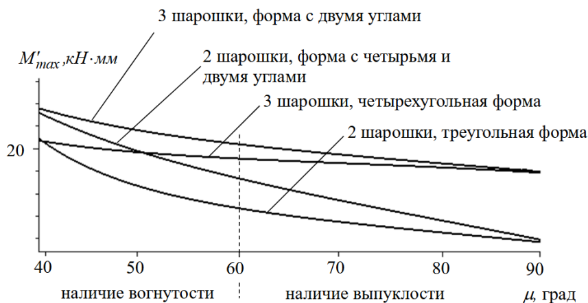
Рис. 3. Максимальные значения крутящего момента M'_{max} в зависимости от формы поперечного сечения скважины, угла \mu и количества шарошек при S=0 , \gamma=15^\circ и площади поперечного сечения скважины, соответствующей площади круглого поперечного сечения скважины диаметром 216 мм (значения при пропорциональности силы сопротивления перекачиванию шарошек длине линии их контакта с забоем 1H=1\text{ мм} )
