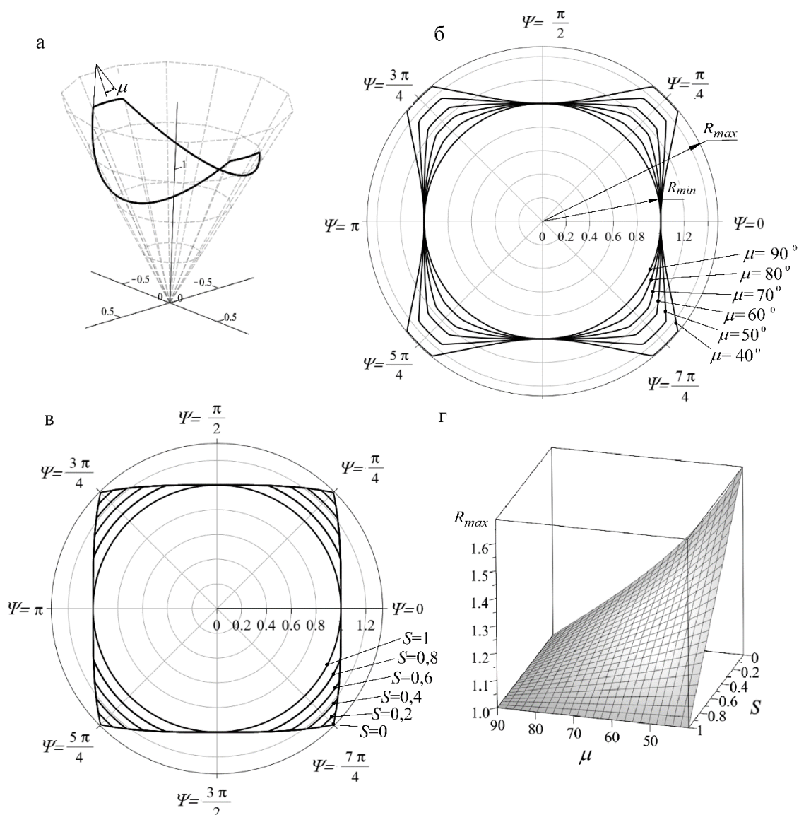
Рис. 1. Влияние формы калибрующей кромки шарошки (а), угла \mu наклона секущей плоскости (б, при S=0,3 ) и степени скругления углов S поперечного сечения (в, при \mu=60^\circ ) на максимальный радиус R_{max} некруглого поперечного сечения (г) при единичном радиусе вписанной него окружной R_{min}=1 и четырехугольной скважине
