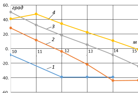
Рис. 3. Влияние координат ковша и разгрузочного каната на угол наклона днища ковша
