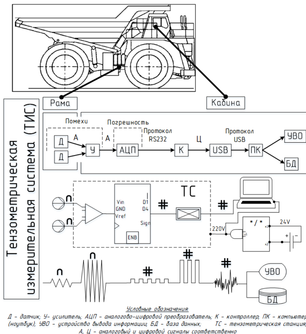
Рис. 2. Принципиальная схема тензометрической измерительной системы (ТИС) Fig. 2. Schematic diagram of a strain gauge measuring system (SGMS)
