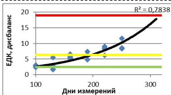
1) прогноз для дисбаланса ротора сетевого двигателя
