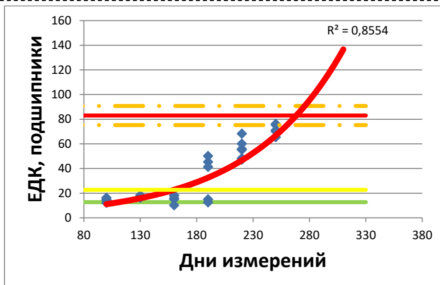
Рис. 6. Среднесрочный прогноз выхода из строя подшипника электродвигателя ленточного конвейера Л-800
