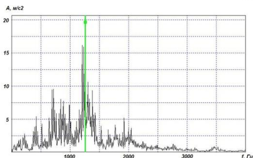
Рис. 2. Спектры вибрации, содержащие признаки наличия основных дефектов энерго-механического оборудования ленточных конвейеров
