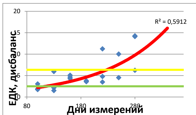
Рис. 5. Среднесрочное прогнозирование развития неуравновешенности ротора ленточного конвейера Л-800
