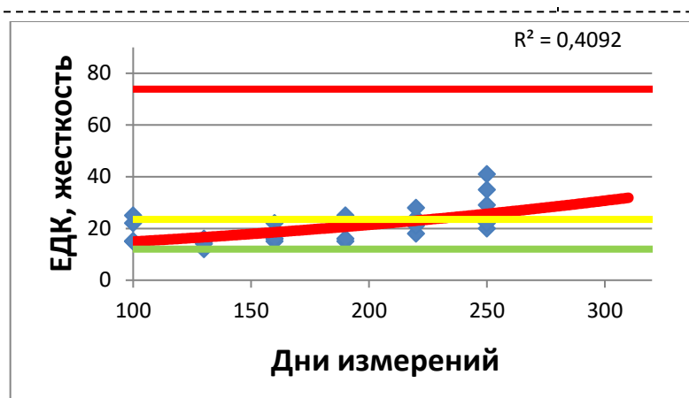
Рис. 3. Среднесрочный прогноз по модифицированному критерию нарушения жесткости системы привода ленточного конвейера Л-800 Fig. 3. Medium-term forecast for the modified criterion of violation of the rigidity of the drive system of the L-800 belt conveyor
