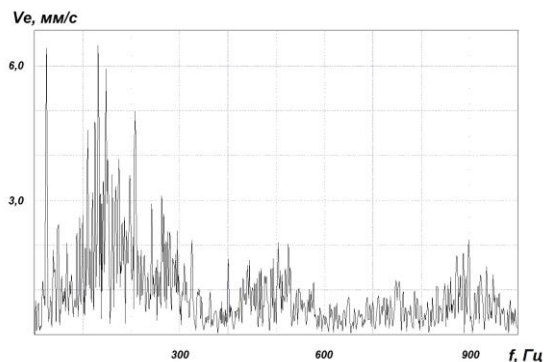
Б) Несоосность валов, локальный абразивный износ зубчатых зацеплений редуктора Misalignment of shafts, local abrasive wear of gears of the gearbox
