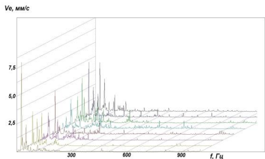
А) Нарушение центровки электродвигателя с редуктором, незначительное нарушение жесткости опорной системы
