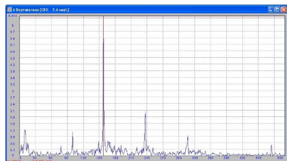
Рис. 9. Спектр виброскорости, характеризующий пульсацию потока воздуха
