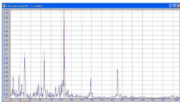
Рис. 8. Спектр вибрации переднего подшипника электродвигателя с присутствующими 2-ой и 3-ей гармониками и ярко выраженной вибрацией на частоте 2 \times f_{cm} .
