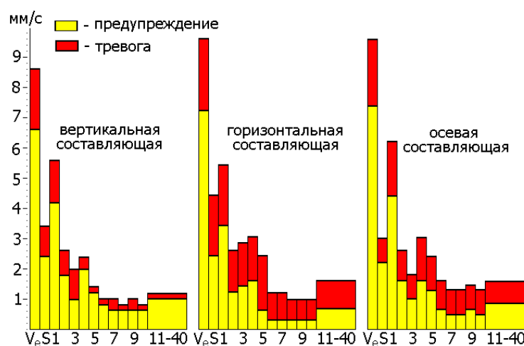
Рис. 6. Нормирование вибрации для осевых вентиляторов типа ВОД и ВОКД
