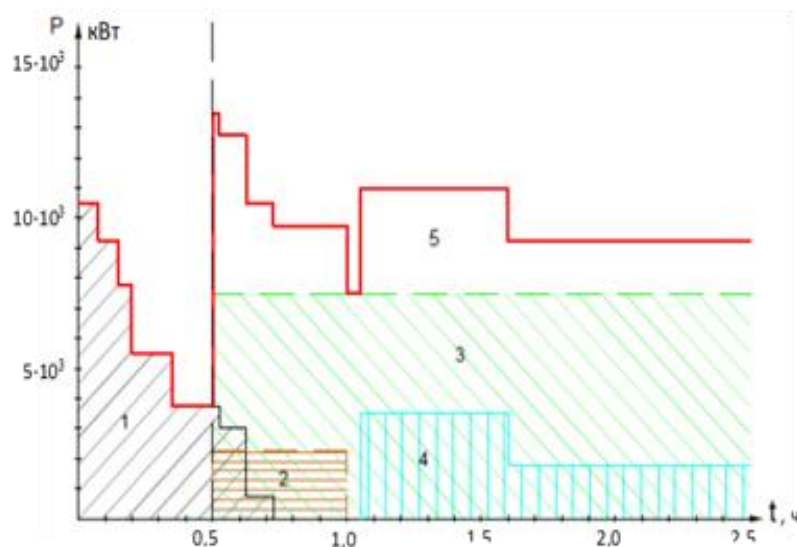
Рис. 4. График формирования технологической и аварийной брони угольной шахты:
