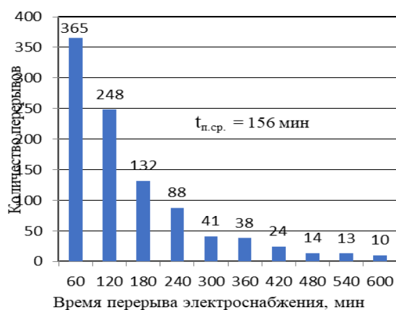
Рис.6. Время перерыва внешнего электроснабжения
