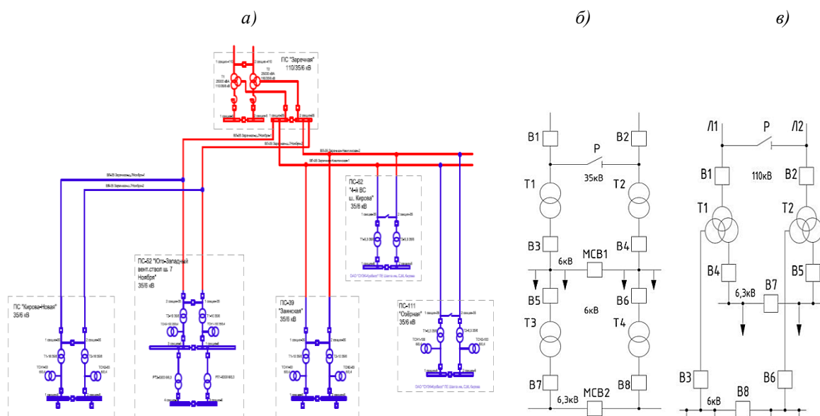
Рис.3 Схемы подключения подстанций угольных шахт к электрическим сетям АО «Кузбассэнерго-РЭС» Fig.3 Diagrams of connection of substations of coal mines to the electric networks of «Kuzbassenergo-RES»
