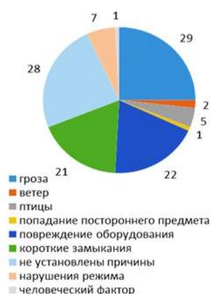
Рис.5. Причины аварий на ВЛ систем электроснабжения угольных шахт
