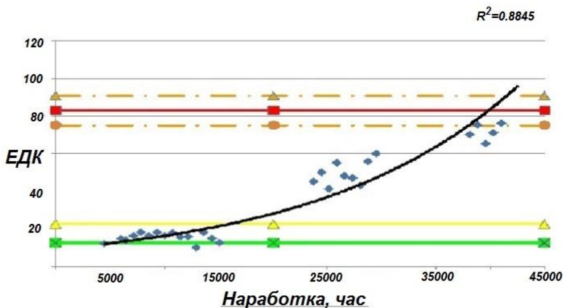
Рис. 1. Прогноз технического состояния подшипника генераторной группы экскаватора ЭКГ-5А Fig. 1. Forecast of the technical condition of the generator group bearing on the EKG-5A type mining shovel
